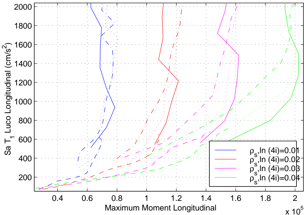
Intensity Measure vs Demand Measure (IDA) - Eq1(-), Eq2(-), Eq3(--), Eq4(:)
